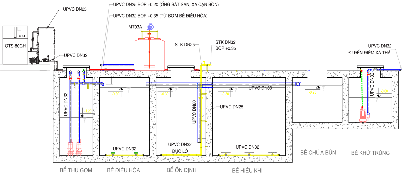
Sơ đồ lắp đặt máy Ozone OzoneTech OTS xử lý nước thải sản xuất dược phẩm công suất 20m3/ngày đêm
