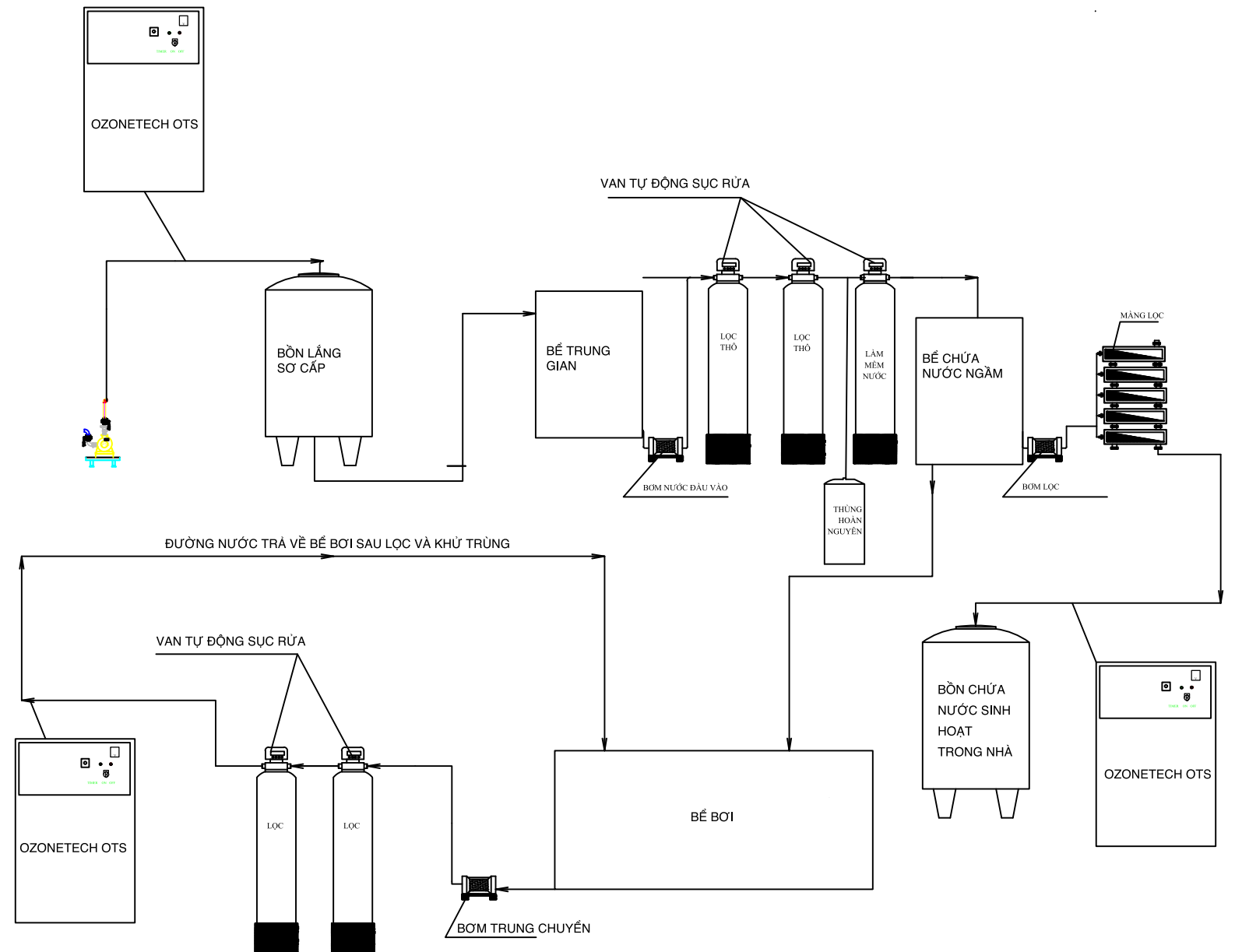
Sơ đồ xử lý nước giếng khoảng 3 - 5m3/h cho biệt thự
